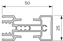
Profilo verticale strutturale aperto Open vertical structural profile
