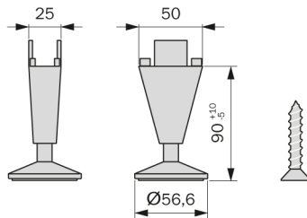
Kit elemento di regolazione Adjustable element kit
