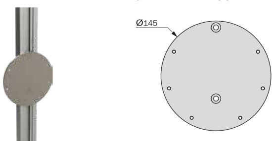
Elemento di raccordo per sistemi appendiabiti saliscendi Wardrobe lift connection element
