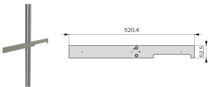
Elemento di fissaggio per telai Frame connection element
