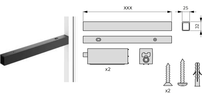
Elemento per appenderia con guarnizione Element for hangers with gasket
