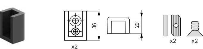
Kit accessori per appenderia Hangers accessories kit
