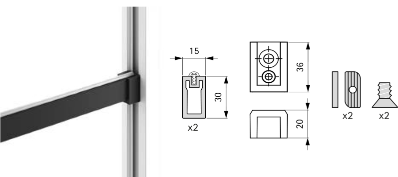
Tubo per appenderia con guarnizione Tube for hangers with gasket
