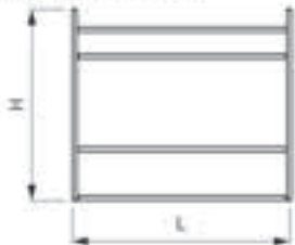
Linea Free unit 3
