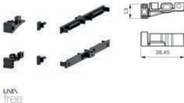
Free κιτ σύνδεσης ραφιών
