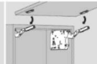
Door Assembly
